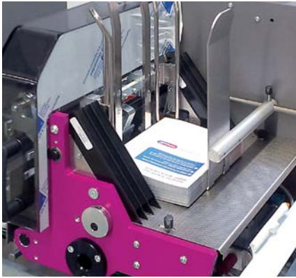
Rotationsanleger RF2
